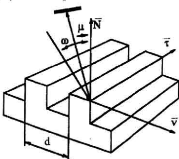
Рис. 4 Падение света под углом на бинарную отражательную квазипериодическую структуру
