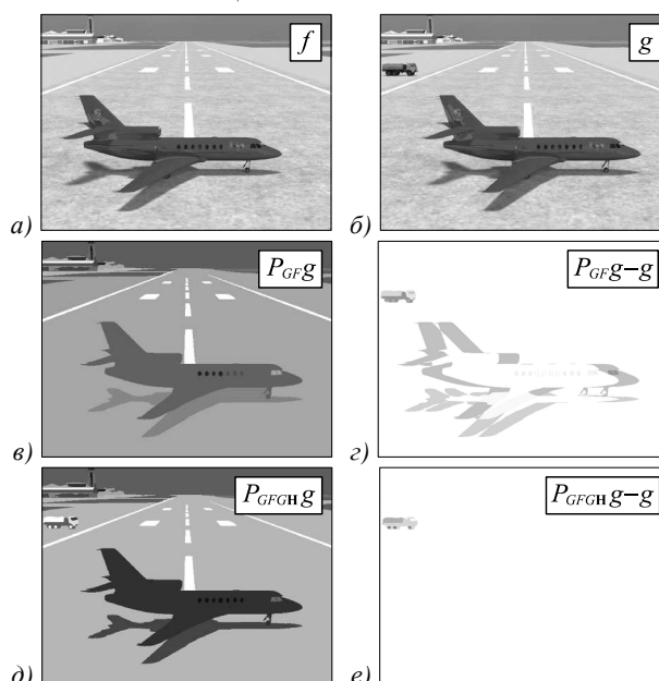
Рис. 1. Выделение отличий в случае изменения геометрии сцены и добавления новых объектов на примере суперпозиции Пытьевских проекторов (в середине) и морфологического выделения отличий на основе референтных EMD-фильтров (внизу): эталонное изображение (а), тестовое изображение (б), суперпозиция проекторов (в), нормализация фона (з), референтный EMD-фильтр (д), нормализация фона (е)
