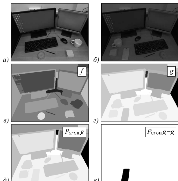
Рис. 2. Морфологическое выделение отличий на основе референтных EMD-фильтров на реальных изображениях: эталонное изображение (а), тестовое изображение (б), сегментированный эталон (в), сегментированный тест (г), референтный EMD-фильтр (д), нормализация фона (е)
