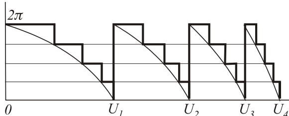
Рис. 2. Квантование цилиндрической линзы по четырем уровням
