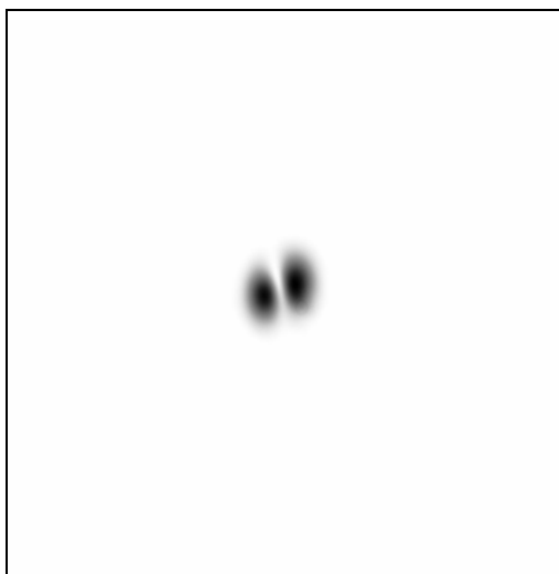
Рис. 14. Распределение интенсивности вышедшего из волокна пучка в дальней зоне
