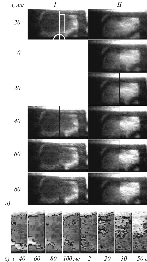
Рис. 6. Визуализация тепловых неоднородностей оптической толщины КГВ во времени
