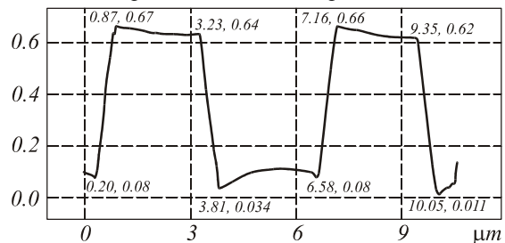
Рис. 5. Профилограмма микрорельефа дифракционной линзы, записанная с помощью сканирующего зондового микроскопа (Ширина зоны: 6,29 мкм.
