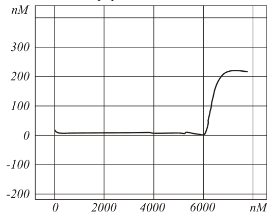
Рис. 4. Профилограмма микрорельефа, представленного на рис. 3
