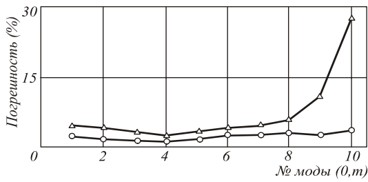
Рис. 2. Среднеквадратичная (▲) и геометрическая (●) погрешности для мод ГЛ, формируемых с помощью фазового ДОЭ с круговой апертурой оптимального радиуса.
