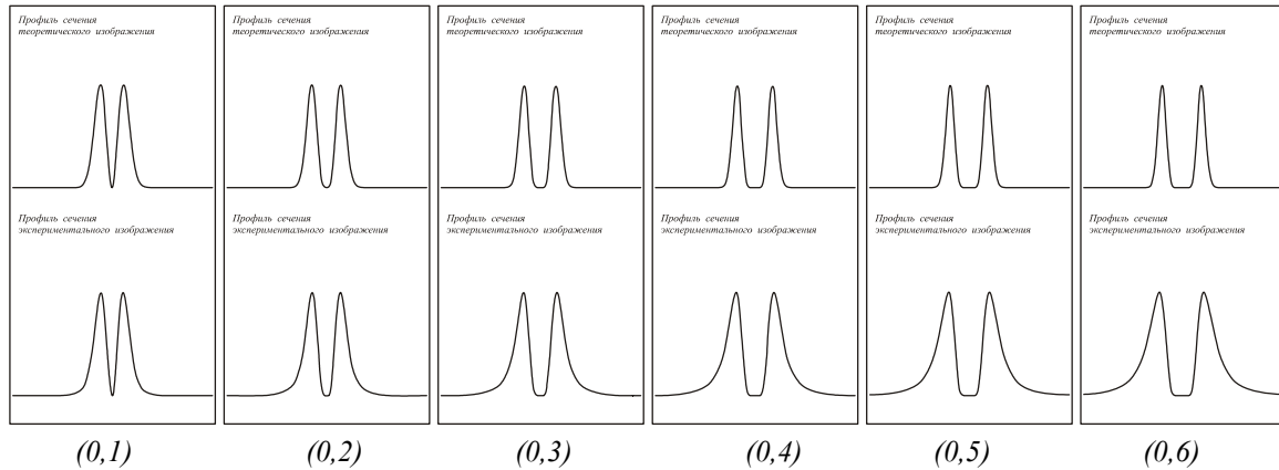
Рис. 3. Поперечные сечения распределений интенсивности мод (0,m) , |m| \leq M для первых 6 мод. Вверху – распределение при использовании АФ ДОЭ, внизу – фазовых ДОЭ.
