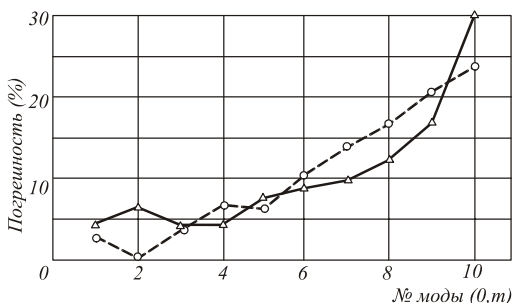
Рис. 4. Среднеквадратичная (▲) и геометрическая (●) погрешности для мод ГЛ, формируемых с помощью фазового ДОЭ, освещаемого гауссовым пучком оптимального эффективного радиуса.
