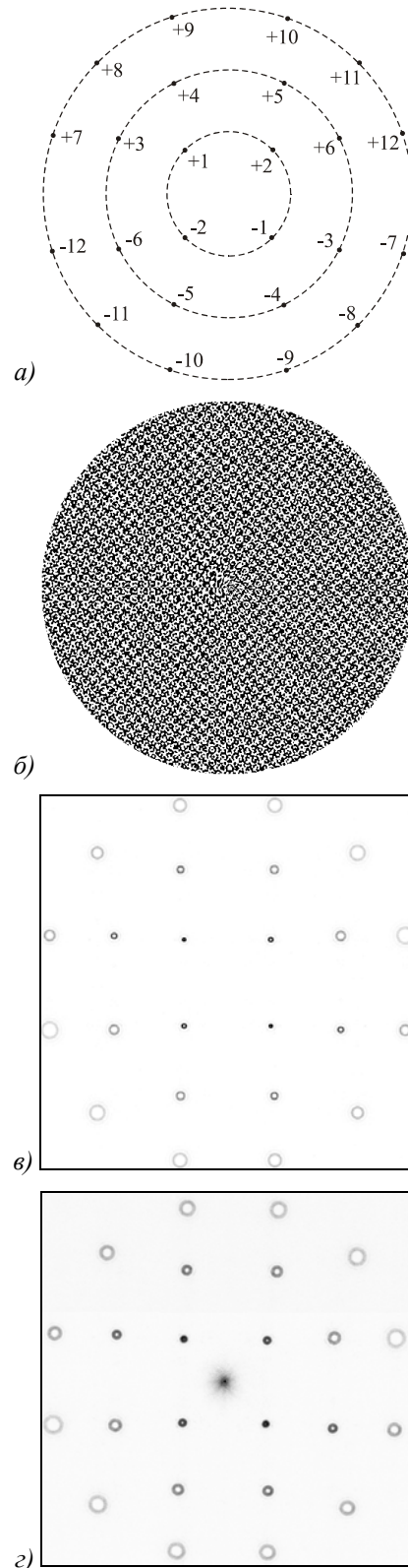
Рис. 7. Схема расположения дифракционных порядков m=\pm 1, \pm 2, \dots, \pm 12 (а) и бинарная фаза ДОЭ (б). Результаты моделирования (в) и эксперимента (г) по формированию винтовых пучков различного порядка в фокальной плоскости линзы.
