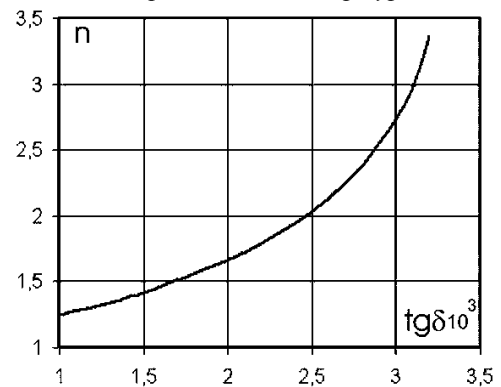
Рис.3. Область оптимальных значений оптических постоянных материала диэлектрика.
