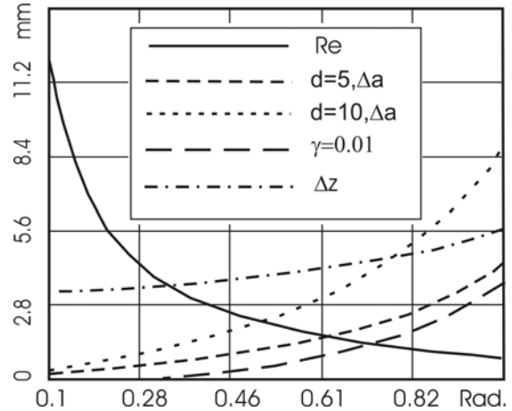
Рис. 5. Зависимость дефокусировки от апертурного угла \alpha оптической системы для n=1,5 :
